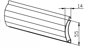
Säleprofiili CD 200
