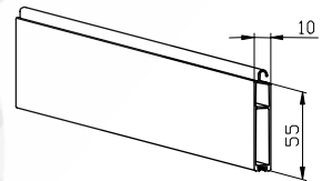
Alasäle 602010
