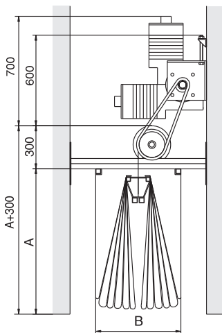
Poimuseinän mitat
