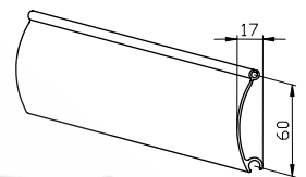
Säleprofiili PX 60
