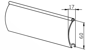
Säleprofiili PX 60
