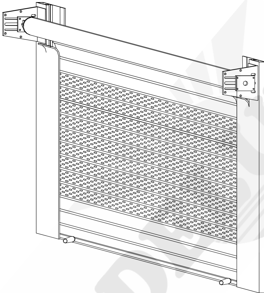
Ohjaukisko 603170
