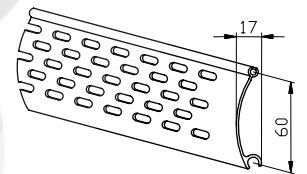
Säleprofiili PX Perfo
