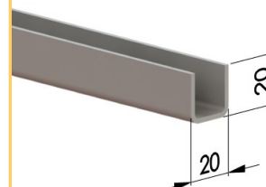
Ohjauskisko U-20x20x2
