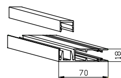
Styrskena 507020
