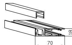
Styrskena 507020
