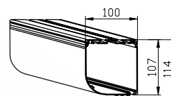
Skyddskåpa PV 105
