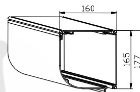
Skyddskåpa PV 160
