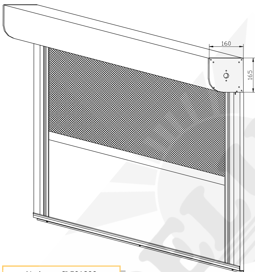
Nedre profil 501300
