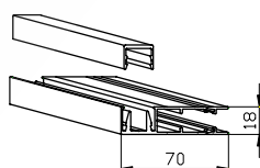
Styrskena 507020
