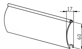
Panelprofil PX 60
