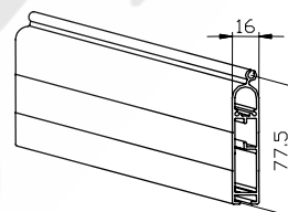
Bottenprofil 606014
