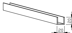
Ohjauskisko U-20x20x20
