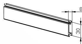
Säleprofiili 603000
