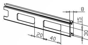
Kalteriprofiili 603040
