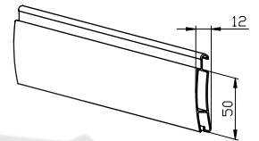
Panelprofil CD 50
