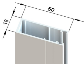
Sivuohjauskisko 505018
