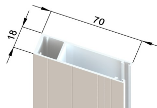
Sivuohjauskisko 507019 (vakio)
