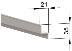
Alaprofiili 501300
