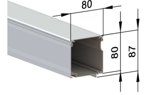
Suojakotelo PV80
