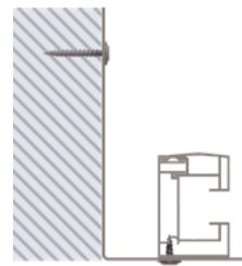
Asennuspelti
