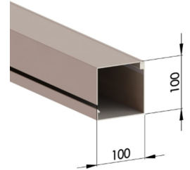
Vetoprofiili 80170037
