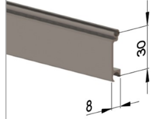
Vetoprofiili 475020
