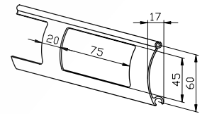
Säleprofiili PX 60-75
