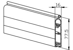
Alasäle 606014
