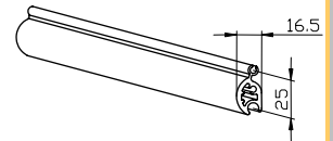
Vahvistusprofiili 606020
