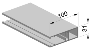
Ohajuskisko 630100
