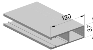
Ohajuskisko 637120
