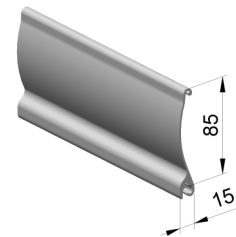
Säleprofiili 608500
