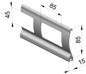
Säleprofiili 608585
